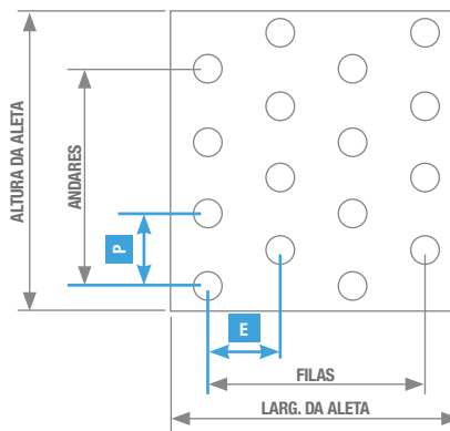
Infraestrutura - Serpentina para água gelada Infraestructura - Serpentina para agua helada
